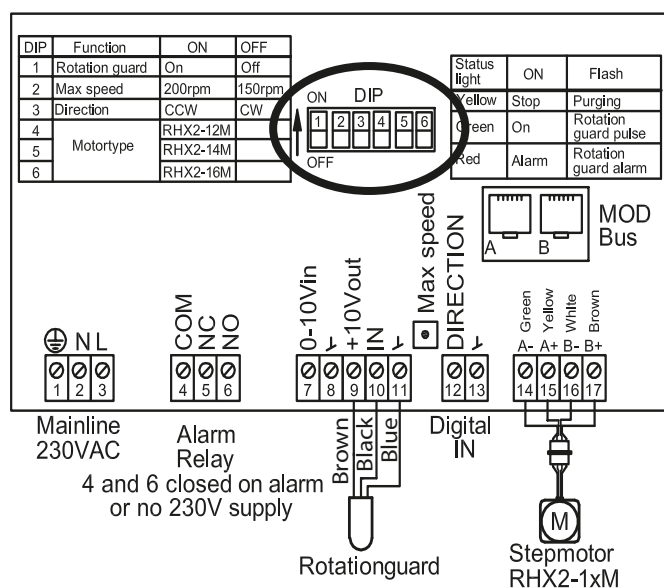
Fig. 2. DIP-omkopplare.
