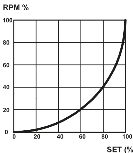
Fig. 3. Kompensering för icke-linjär värmeöverföring.
