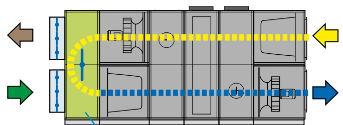
Umluftsektion RX/HC (Zubehör)
