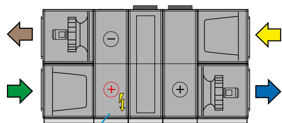
Elektrischer Luftheritzer in RX/HC (Zubehör)
